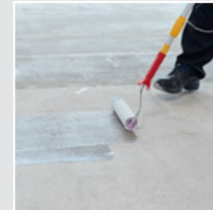
2 Zur Staubbindung und besseren Haftung wird der Estrich grundiert.
