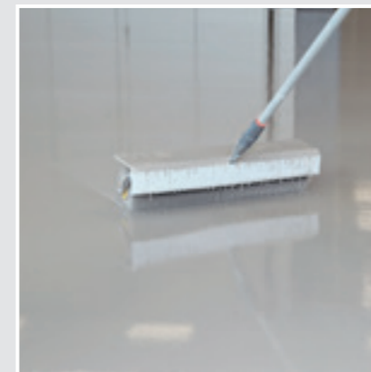
6 Vollflächiges Spachteln des Untergrundes mit SCHÖNOX HS 10. Wir empfehlen die Raketentechnik und das Nachbearbeiten mit einer Stachelwalze.
