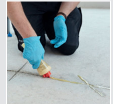
3 Kraftschlüssiges Schließen von Scheinfugen, Rissen und Arbeitsfugen mit SCHÖNOX SGH.
